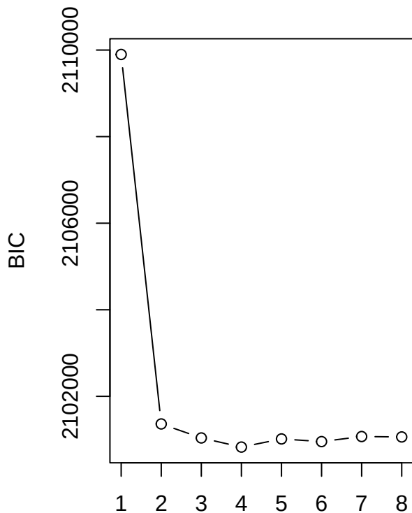
BIC
